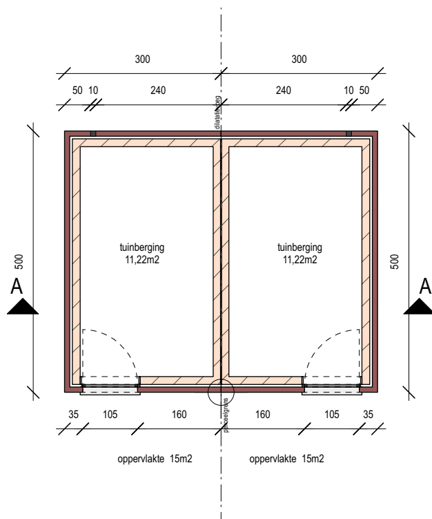
GRONDPLAN BIJGEBOUW 1:100 lot 1 lot 2
